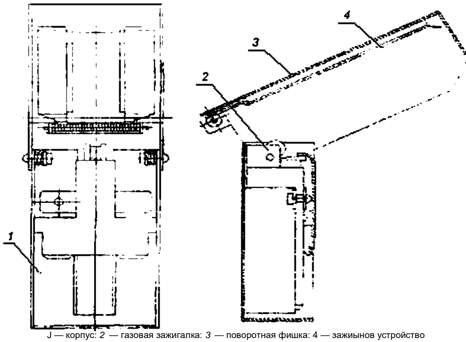
Рисунок Д.1 — Схема малогабаритного переносного прибора для оценки качества огнезащитной обработки деревянных конструкций
