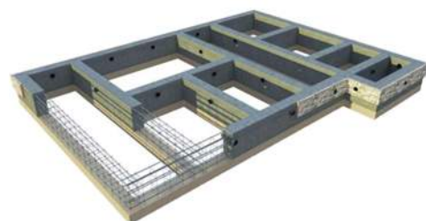
ФУНДАМЕНТНЫЕ РАБОТЫ
