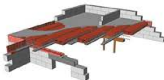
ЖЕЛЕЗОБЕТОННЫЕ КОНСТРУКЦИИ
